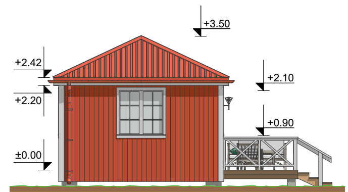
FASAD D
