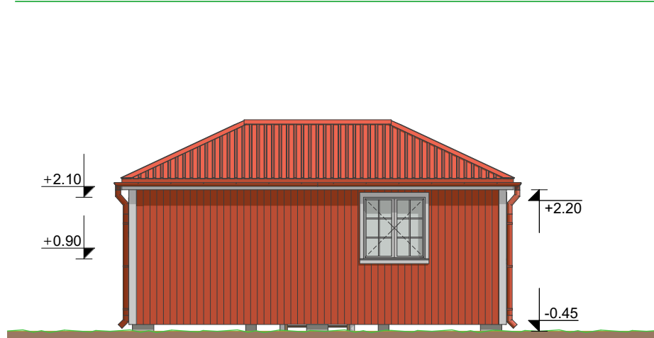
FASAD B
