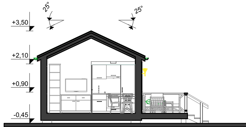
Sektion S-07
